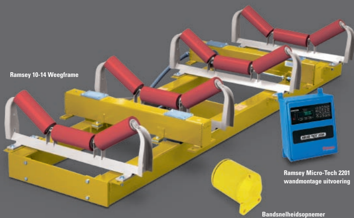
Bandsnelheidsopnemer
